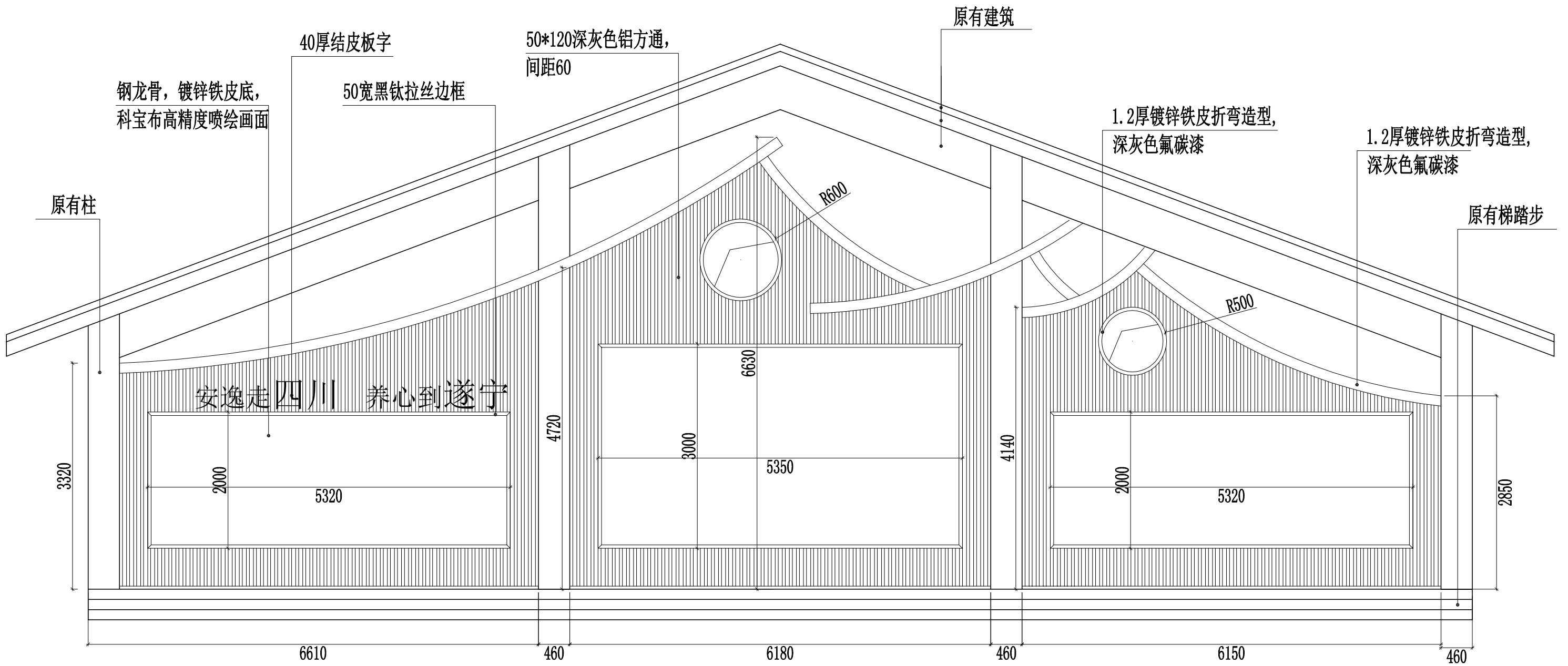
遂宁西服务区文旅宣传栏立面图
